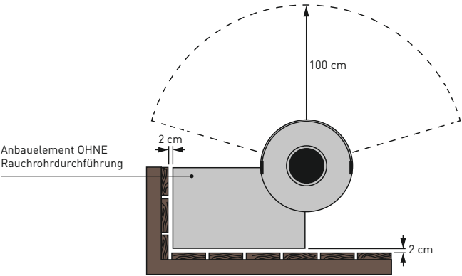
Draufsicht Brennkammer
