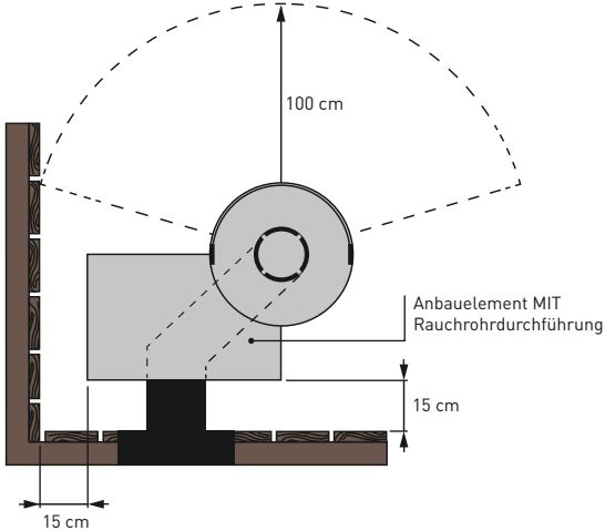
Draufsicht Brennkammer
